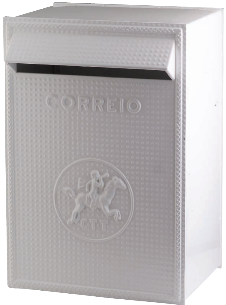
CAIXA CORREIO | REF. ML 307 MED. G 410x280x200 c/porta à frente ou atrás MED. M 300x340x200 c/porta atrás MED. P 220x280x200 c/porta atrás
